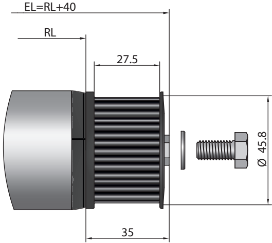
M8 内螺纹紧固装置
