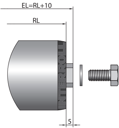
M8 内螺纹紧固装置
