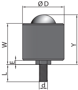
螺纹销
