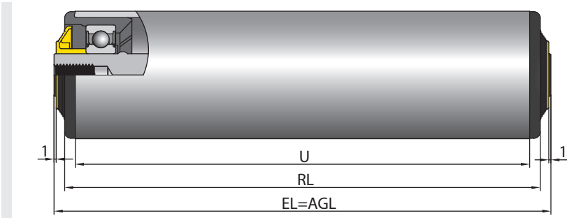
滚筒，直径 60 mm，带聚酰胺轴承座
