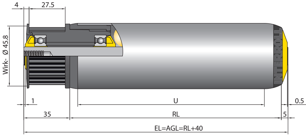
同步带驱动头 (8 间距和 18 齿)
