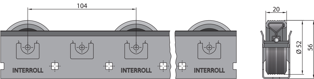
带 2200 系列滚轮的轨道，带橡胶垫圈
