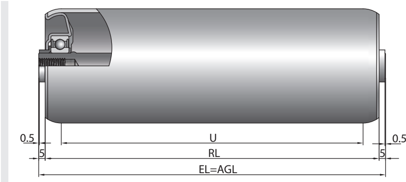
滚筒，直径 80 和直径 89 mm，带钢制轴承座
