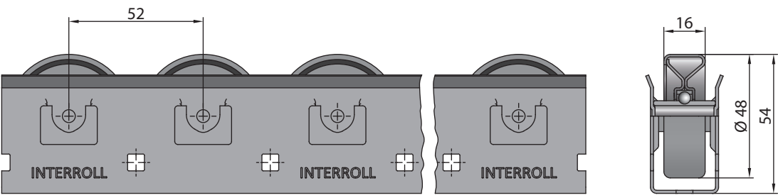
带 2130 系列滚轮的轨道，带橡胶垫圈
