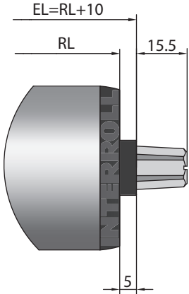
锥形六角弹簧轴
