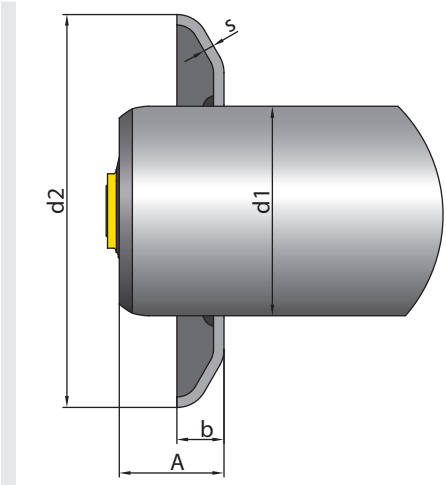
图：左法兰
